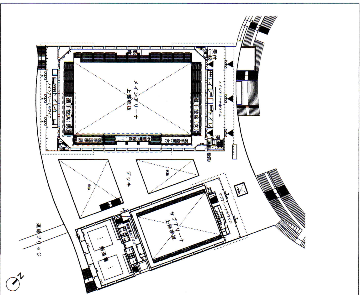
2階平面図
