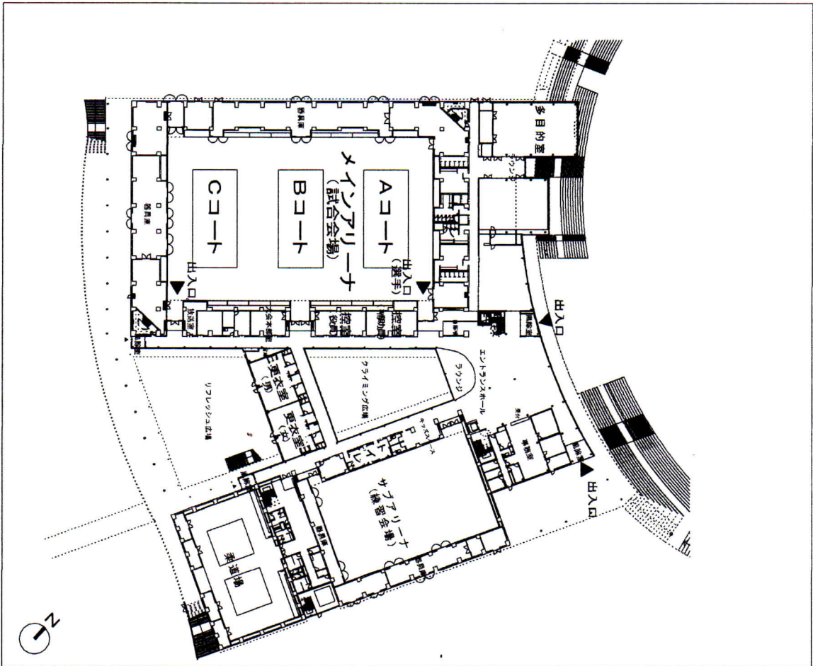
1階平面図
